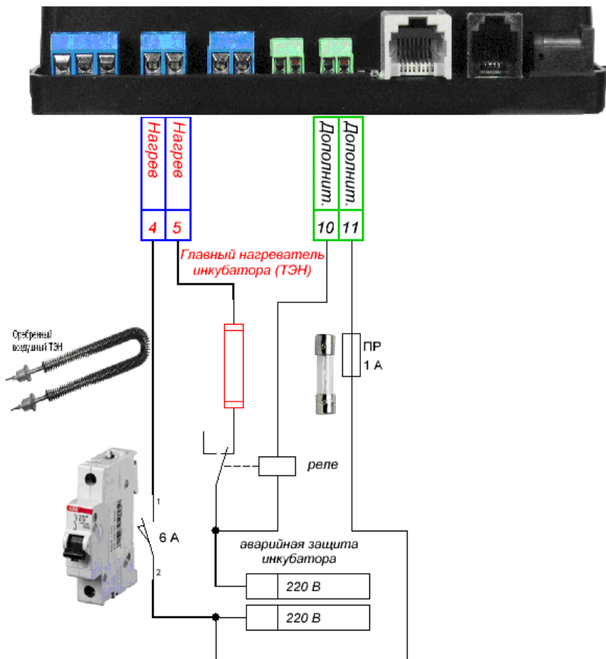
Схема защиты от пробоя симистора.
